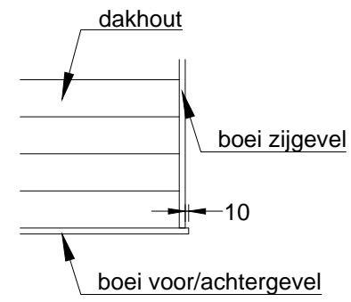
Bovenaanzicht aansluiting boeien
